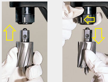
刀具安装/刃物の取り付け
