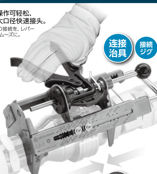
图片是SP快速接头Type A (16SP-A) 写真はSPカップType A/16SP-A (Rc2)
