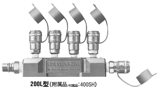
200L型(附属品/付属品:400SH) (本品标准配置有防尘罩。) (本品は防塵キャップを標準装備しています)
